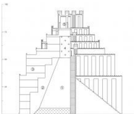
Abbildung 3: Zikkurat von Babylon, Aufbau nach Hartmann [29] 1. Kernmassiv teilweise erhalten, 2. Lehmziegelmantel, 3. Ziegelmauerwerk, 4. Füllungen des Nebukadnezar, 5. Hochtempel Bildurheberrechte: Pahl, B.; Teichmann, J. nach Hartmann [Lit. 29, S. 111]
